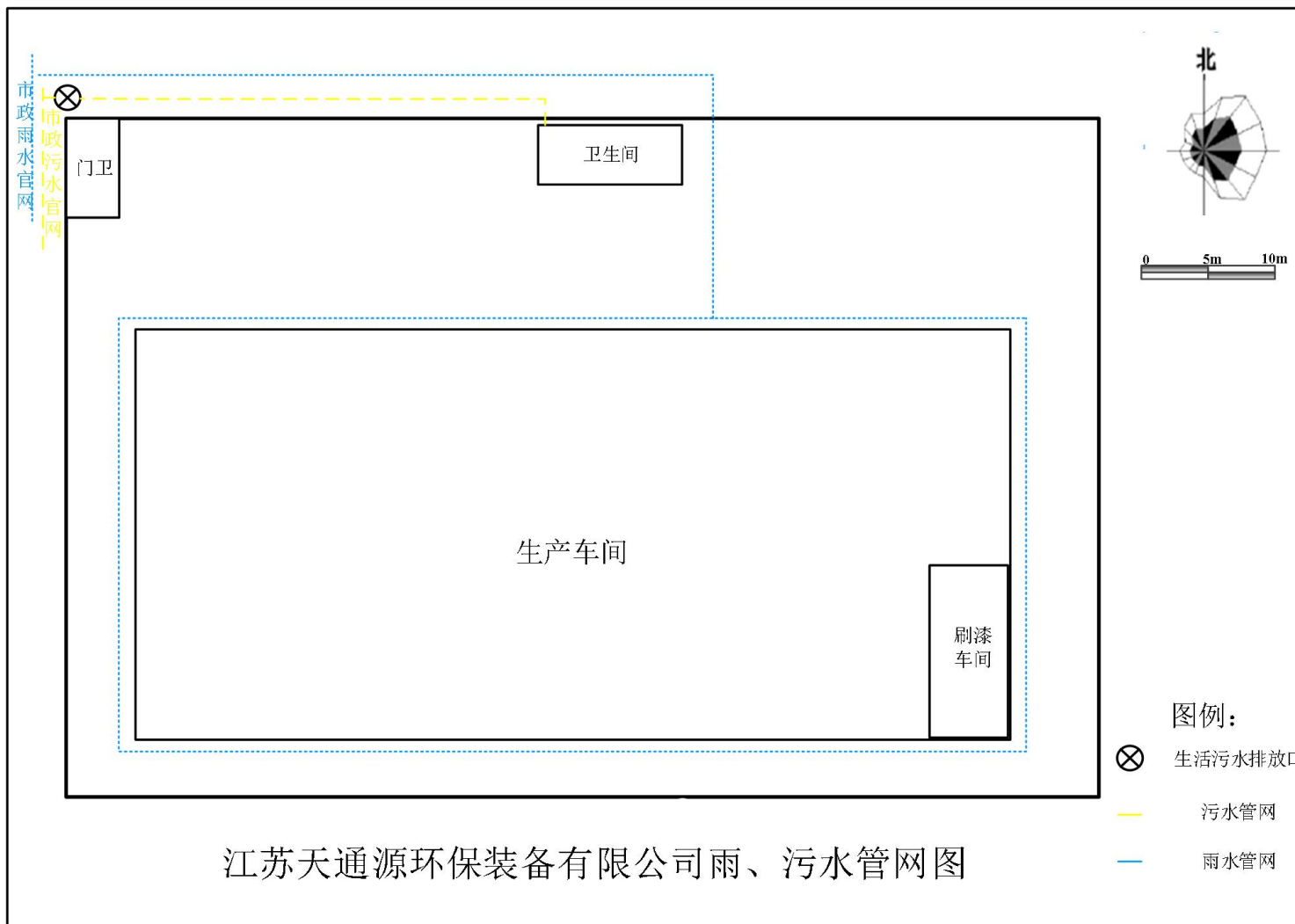
附图 5 雨、污水管网图
